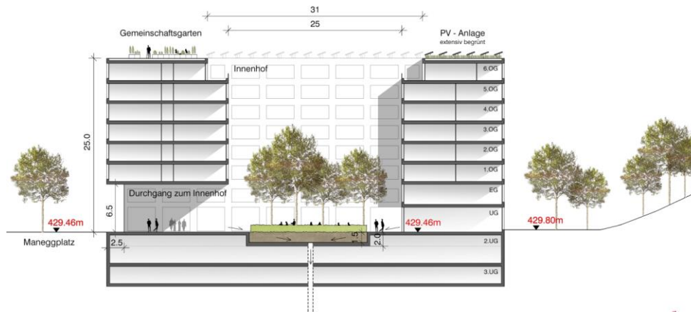
Abbildung 1: Systemschnitt Ost-West Machbarkeitsstudie Seniorenresidenz Green City, Zürich Die Grundrisszeichnungen befinden sich im Anhang A1.
