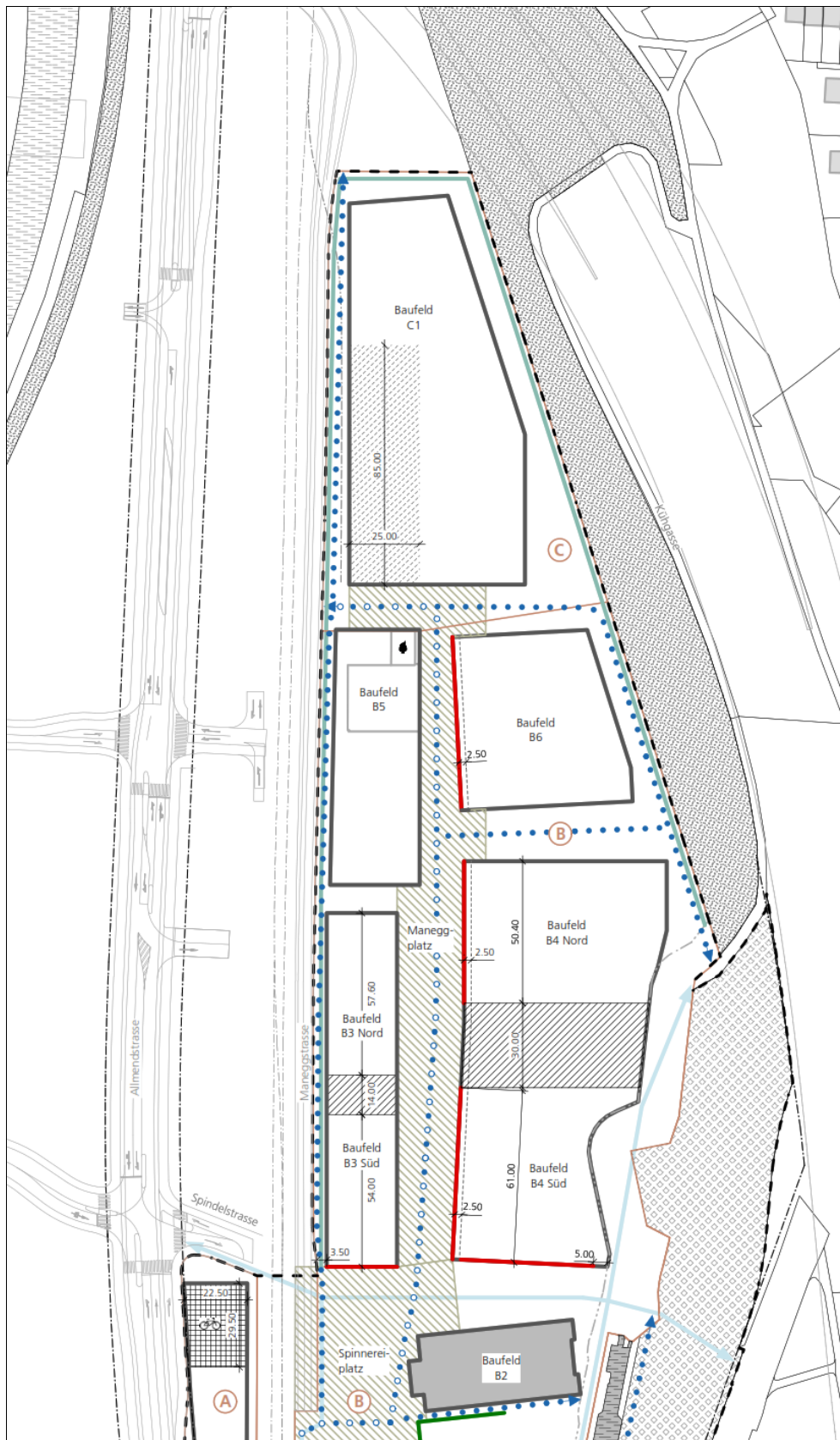
Abbildung 2: Situation (Ausschnitt) aus dem ergänzenden privaten Gestaltungsplan «Green City.Zürich» (2012) [2]
